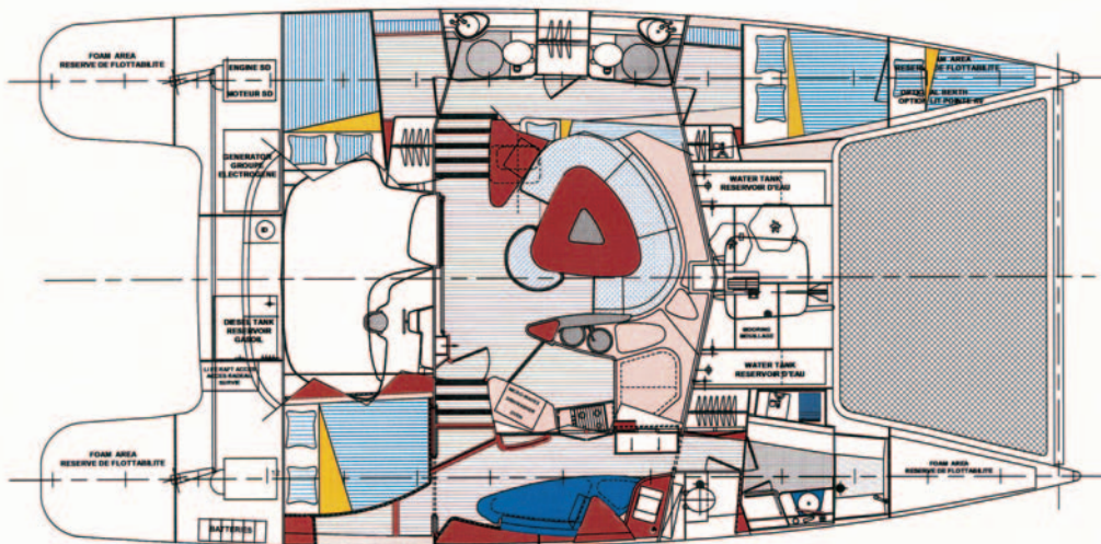
BAHIA 46 Maestro
